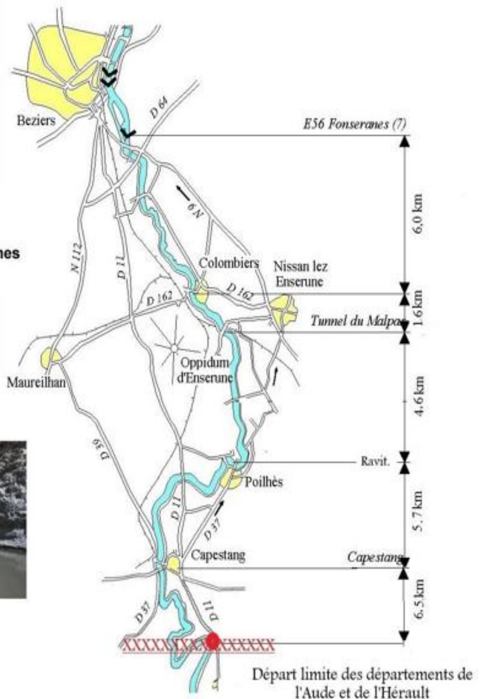
Tunnel du Malpas (1679-1680)
